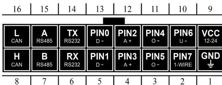
Рисунок 1 – Распиновка разъёма
