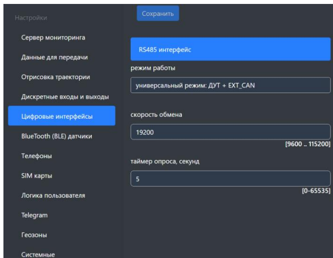
Рисунок 7 - Настройки RS485
