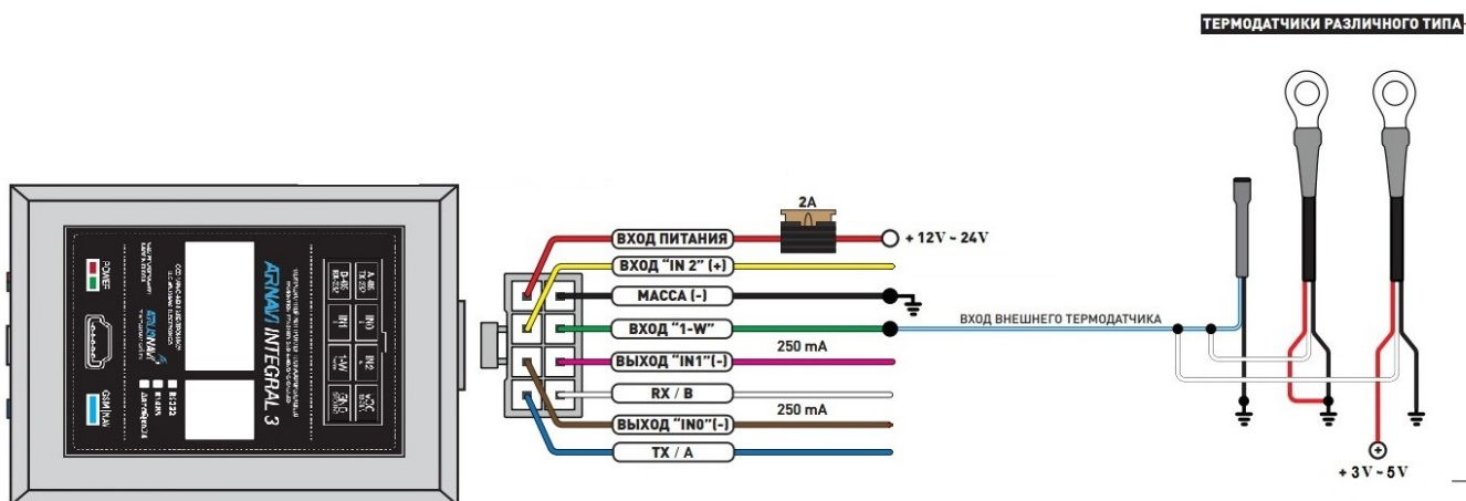
Схема подключения термодатчиков
