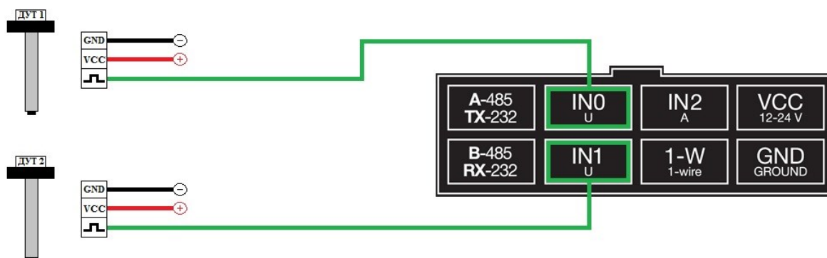
Схема подключения частотных ДУТ
