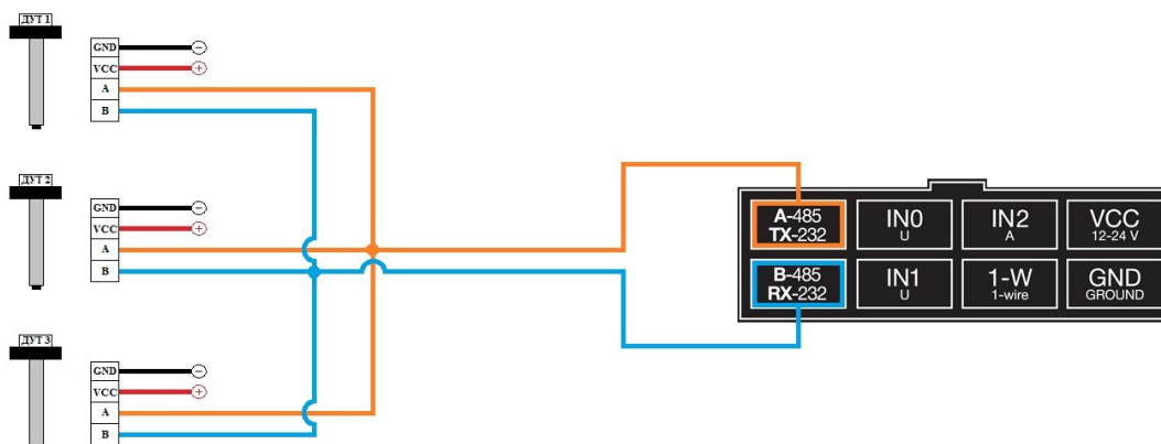
Рисунок 28 – Схема подключения нескольких ДУТ по RS485
