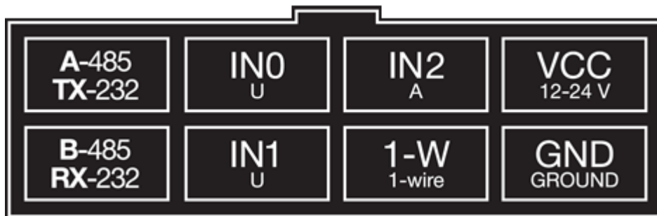
Распиновка основного разъёма
