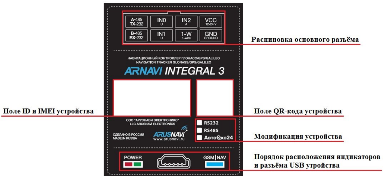
Информационная часть устройства
