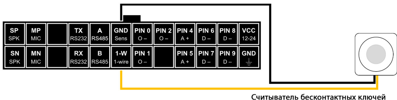
Рисунок 9 - Схема подключения считывателя бесконтактных ключей
