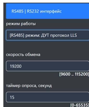
Рисунок 7 - Настройки RS485 | RS232
