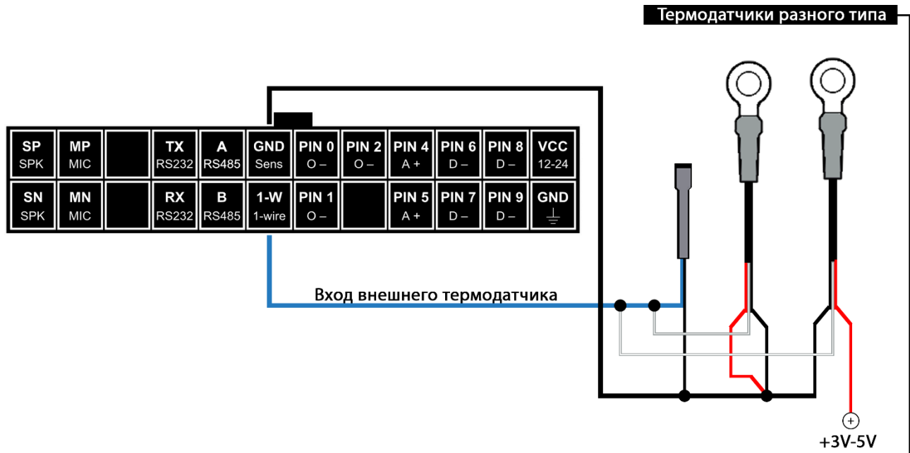
Рисунок 8 - Способы подключения термодатчиков
